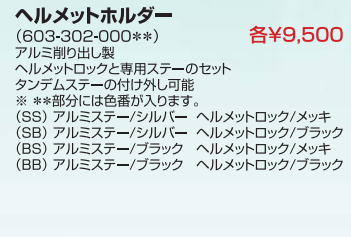
リアアクスルプロテクター ¥11,500 (345-302-000) プロテクターサイズ: φ60 ジュラコン製 アルミ削り出し製 ※方が一の転倒時に、アクスルシャフト部分及び、ブレーキマワリを保護します。
